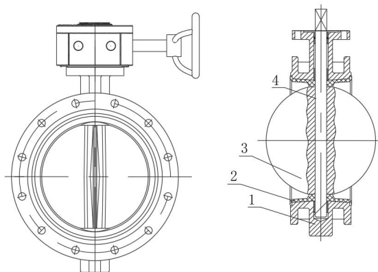
D341X 法兰消防蝶阀结构图
