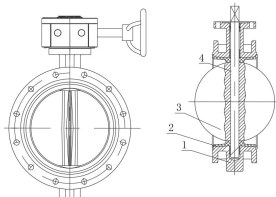
D341X 法兰消防蝶阀外形尺寸图
