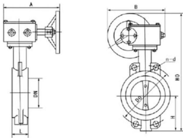
D371X 涡轮对夹蝶阀外形尺寸图
