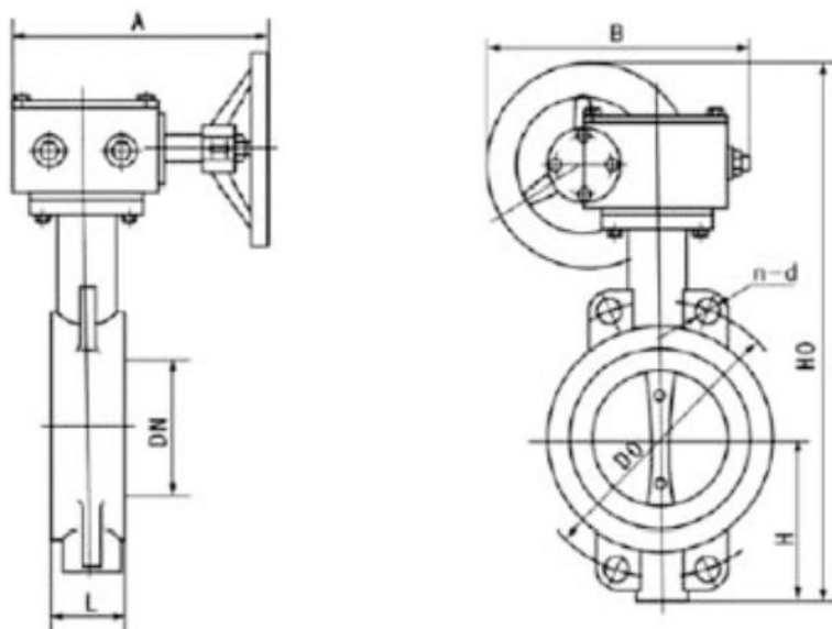
D371X 蜗轮对夹蝶阀结构图
